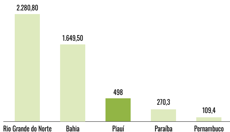
FIGURA 25 - NOVOS PARQUES EÓLICOS (SOMA DA POTÊNCIA - MW)
