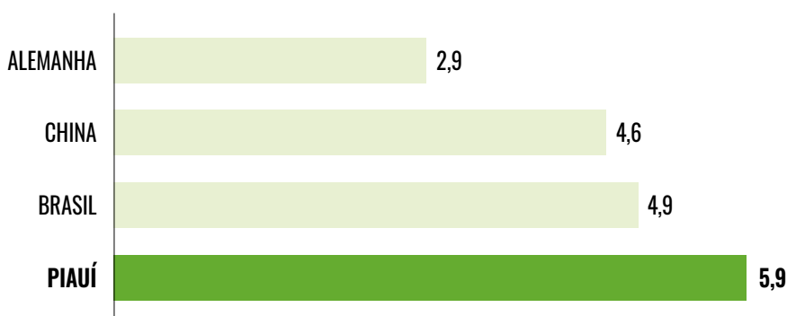
FIGURA 23 - MÉDIA ANUAL DA POTÊNCIA DE IRRADIAÇÃO SOLAR
