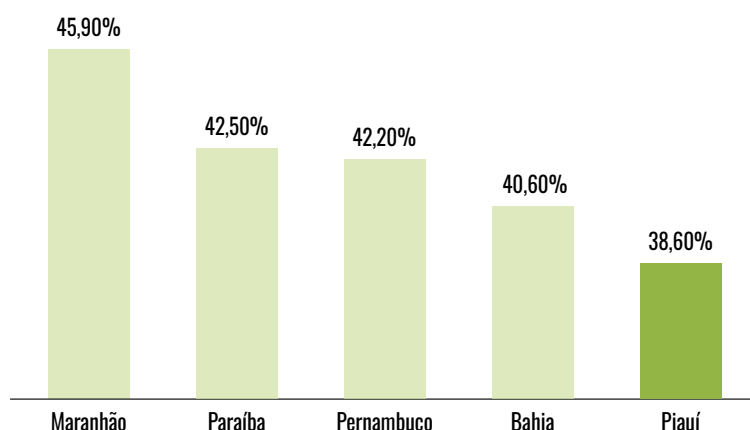
FIGURA 26 - FATOR DE CAPACIDADE MÉDIA POR ESTADO
