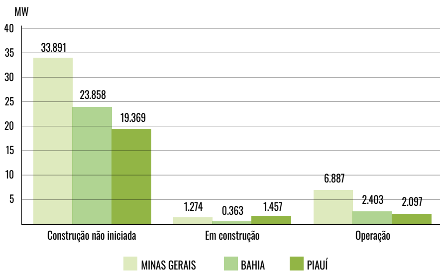
FIGURA 24 - GC PARA CAPACIDADE INSTALADA DE USINAS SOLARES
